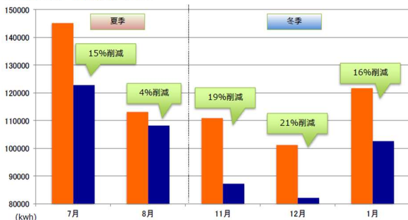
●夏季/冬季 電気使用量グラフ
